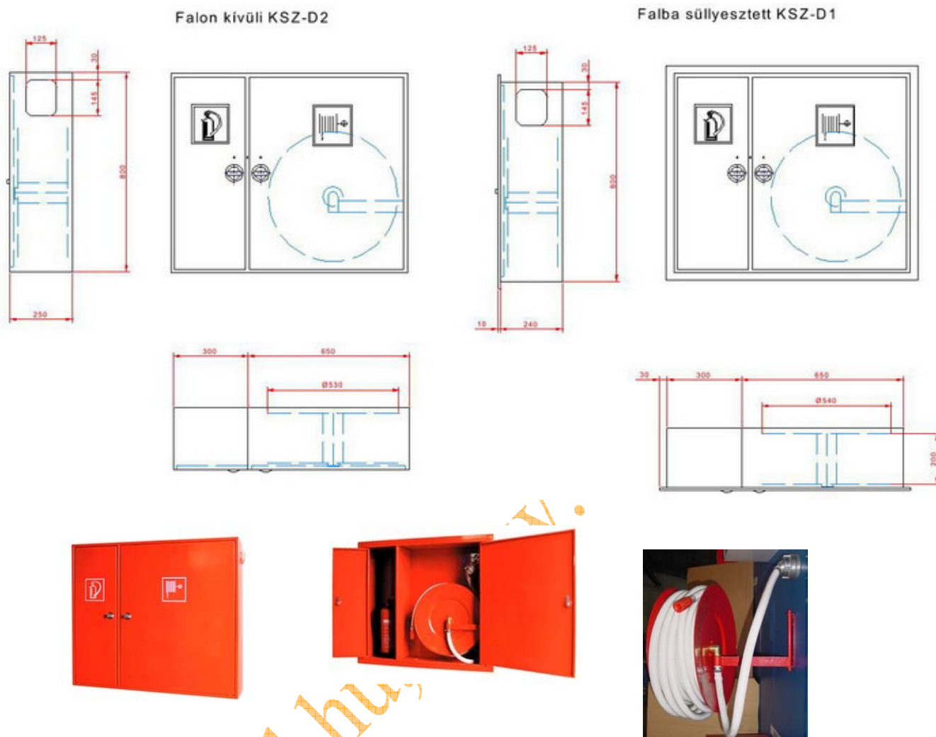
Kombinált tűzcsapszokrény KSZ-D2 falon kívüli / out of the wall
